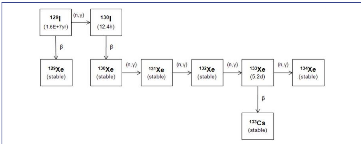
| I-129 핵종변환(I-130) |
